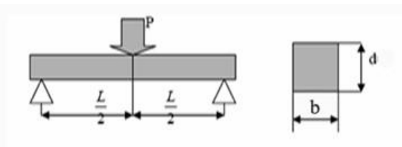
Gambar 1. Penampang uji bending
