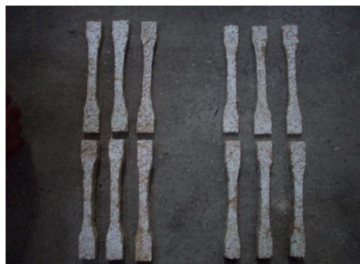
Gambar 4. Spesimen uji Impak komposit sekam padi bermatrik urea formaldehyde
