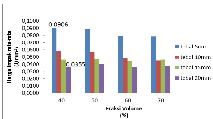
Gambar 7. Grafik Hubungan Kekuatan Impact Rata-rata dengan Fraksi Volume.
