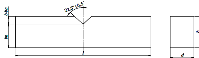
Gambar 2. penampang uji impak
