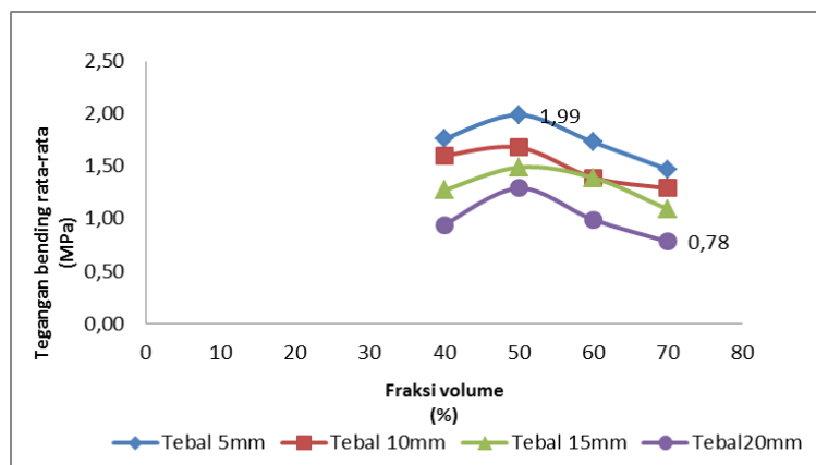
Gambar 6. Grafik Hubungan Tegangan bending rata-rata dengan fraksi volume
