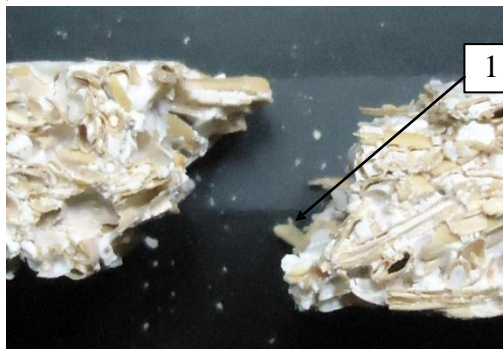
Gambar 9. Foto struktur makro pada spesimen uji Impak.
