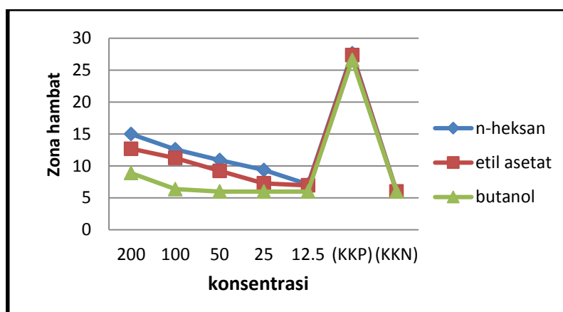
Gambar 3 Grafik Rata-Rata Diameter Zona Hambat Fraksi n-Heksan, fraksi Etil-asetat dan Fraksi Butanol
