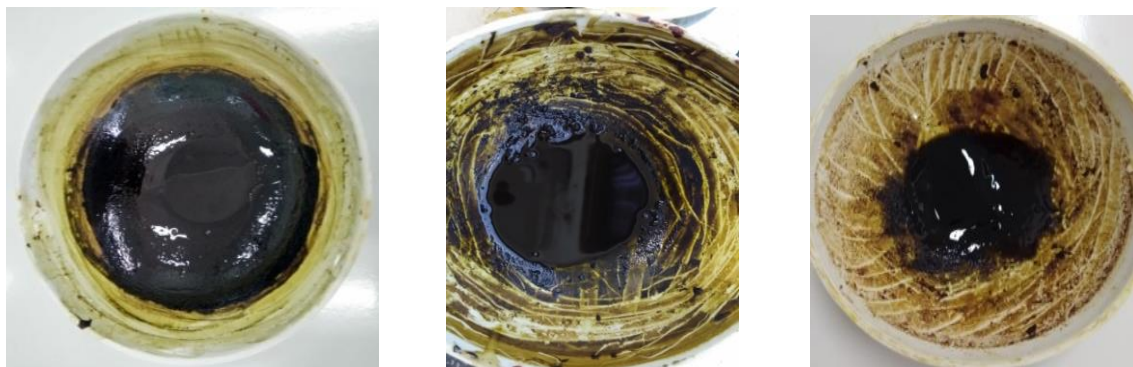
Gambar 2. (a) Hasil Fraksi N-heksan (b) Hasil Fraksi Etil Asetat (c) Hasil Fraksi Butanol
