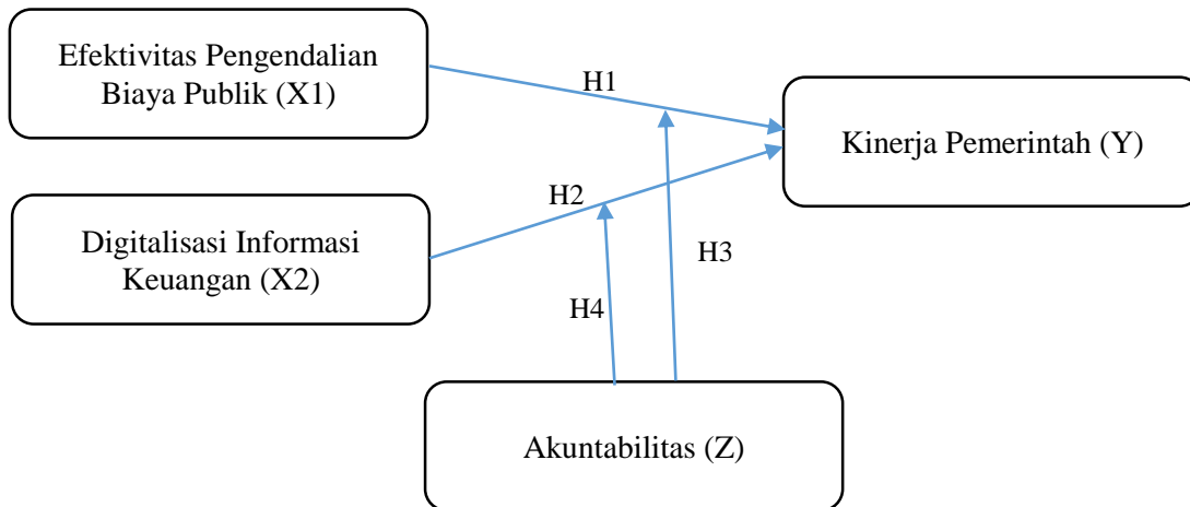
GAMBAR 1. KERANGKA PENELITIAN
