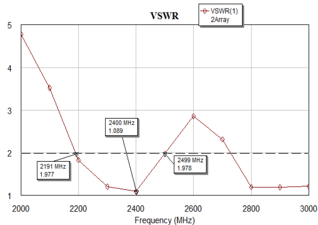
Gambar 5. VSWR antenna dengan susunan peradiasi array 2x2.
