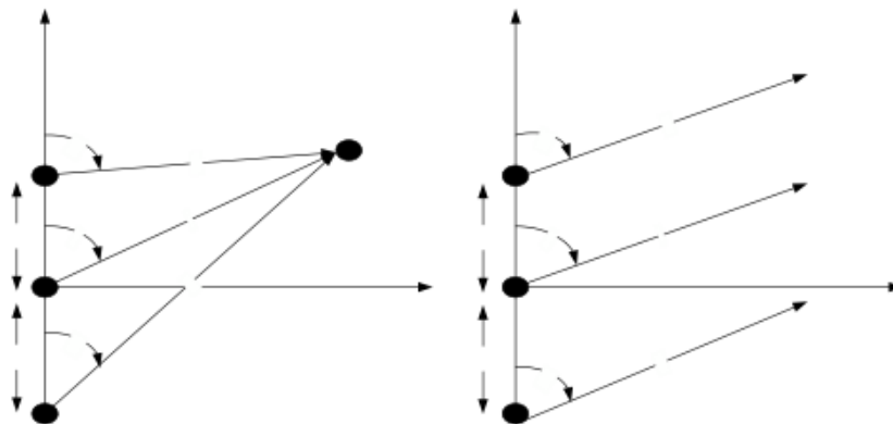
Gambar 2. Geometri Dua Elemen Array [6]
