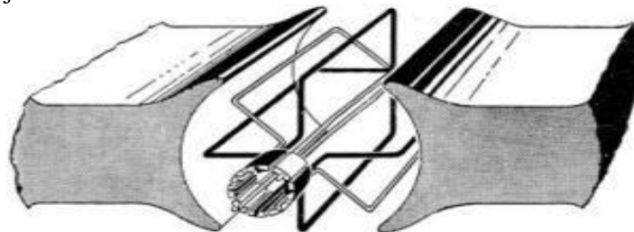
Gambar 3. Skema Generator dengan Empat Lilitan Armature
