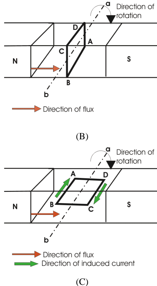
Gambar 3. Prinsip Kerja Generator DC
