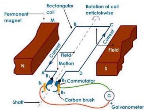
Gambar 2. Skema Bagian-Bagian Generator DC
