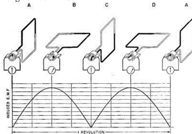
Gambar 2. Grafik Voltase yang Dibangkitkan Generator DC
