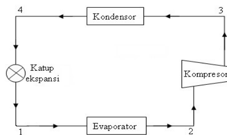
Gambar 2.2. Siklus Kompresi uap
