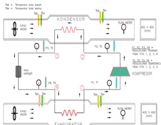
Gambar 3.2 Diagram mesin pendingin kompresi uap
