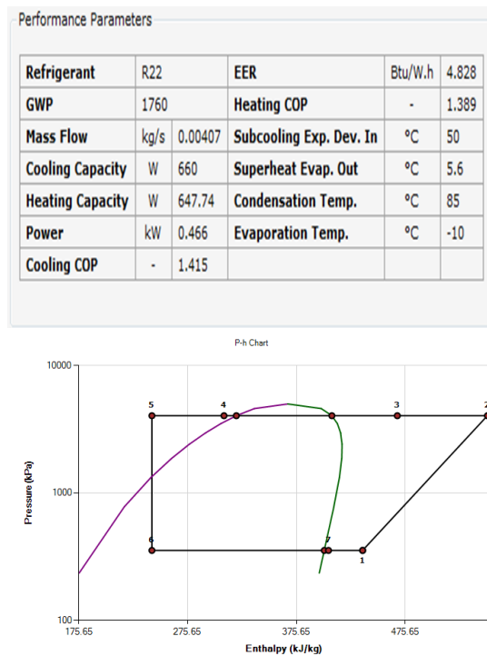
Gambar 4.2 Ph chart dari software genetron properties ketika low fan
