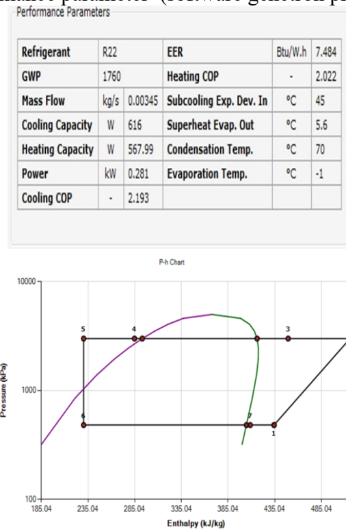
Gambar 4.1 Ph chart dari software genetron properties ketika high fan
