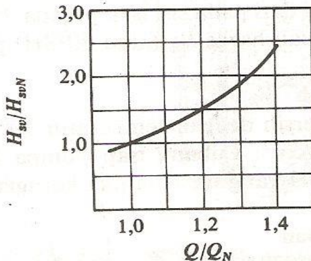
Gambar 3.3 : NPSH yang diperlukan dari titik efisiensi tertinggi ke kapasitas besar.
