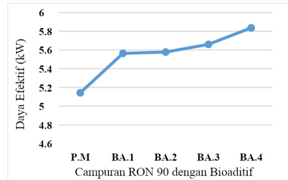
Gambar 2. Grafik daya bahan bakar RON 90 dengan Bioaditif
