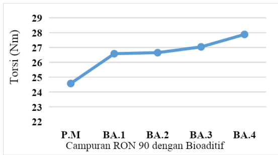
Gambar 1. Grafik torsi bahan bakar RON 90 dengan Bioaditif
