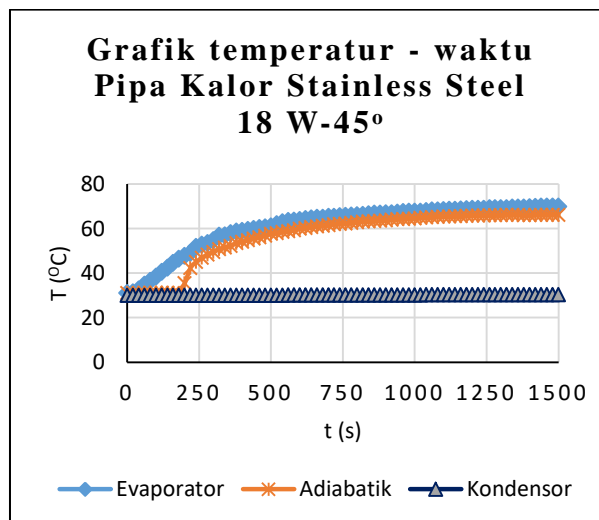
Grafik 6. Pipa kalor beban 18 W- 45°
