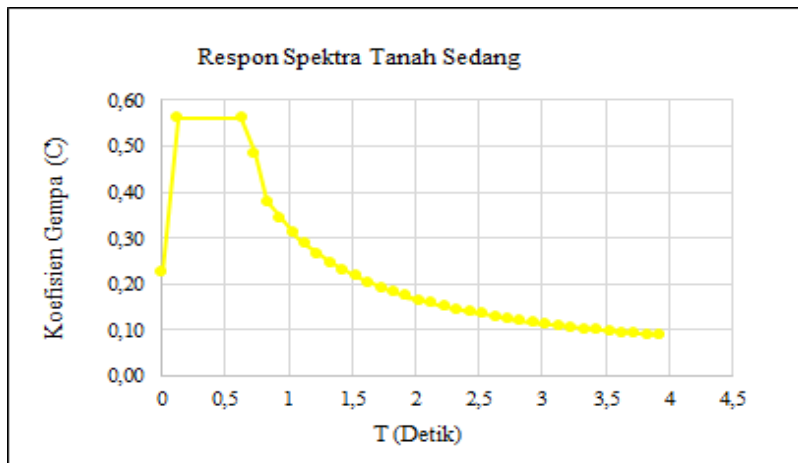
Gambar 3. Grafik Respons Spektrum Sumber: Puskim.co.id
