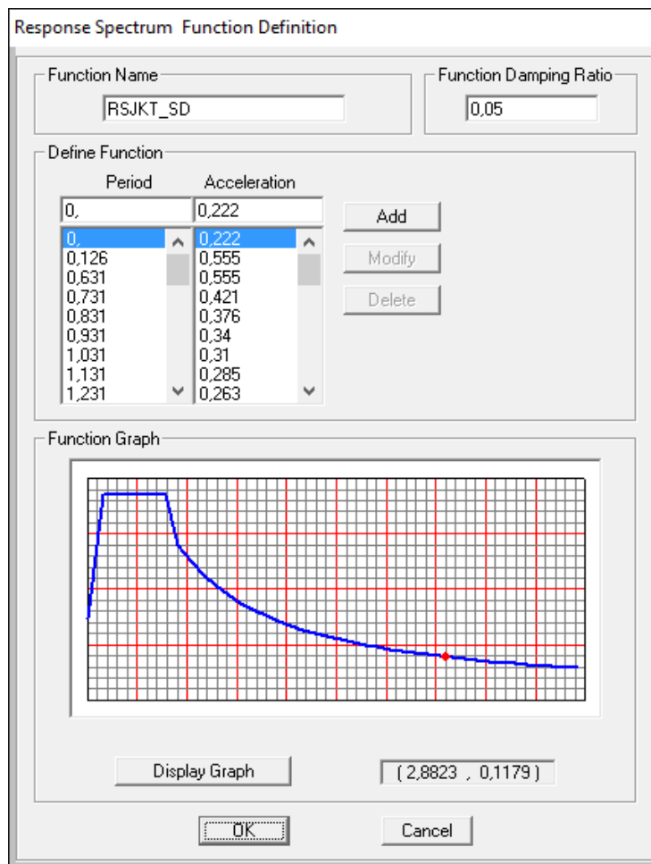
Gambar 4. Data Respon Spektrum
